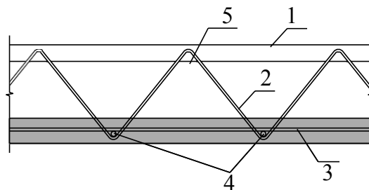
图5.2.8 吊点位置横向分布钢筋与预制底板内钢筋位置关系示意
