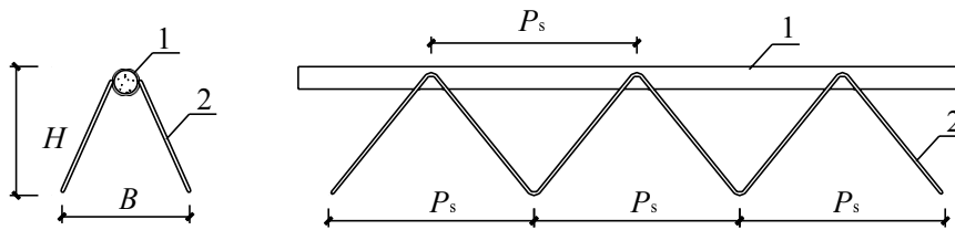
图5.2.1 钢管桁架示意
