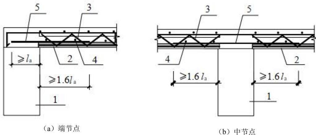
图 5.4.4 无胡子筋板端支座构造示意
