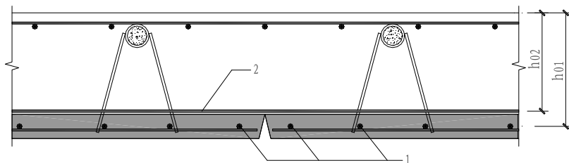
图 5 双向叠合板两个方向截面有效高度示意图
