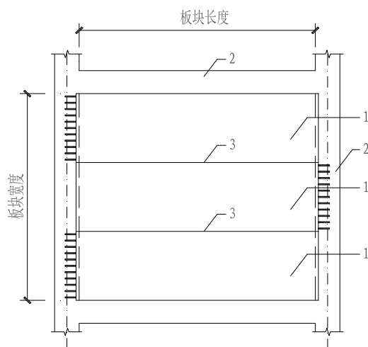
图 4.1.3 叠合板的预制底板布置形式示意
