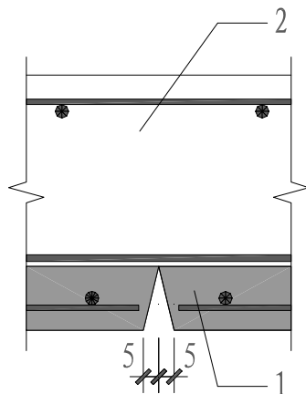
图 5.3.1 钢管桁架预应力混凝土预制底板侧斜平边接缝构造示意
