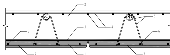
图3 密拼式接缝
