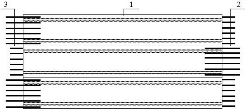
图5.4.2 叠合板设置端部连接钢筋构造 1—预制底板；2—胡子筋；3—端部连接钢筋
