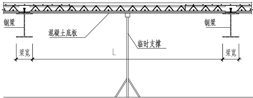
图 10 (b) 与钢梁搭接浇筑叠合层混凝土前设临时支撑示意图
