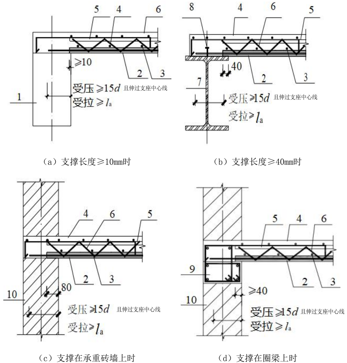
图 5.4.1 板端支座构造示意
