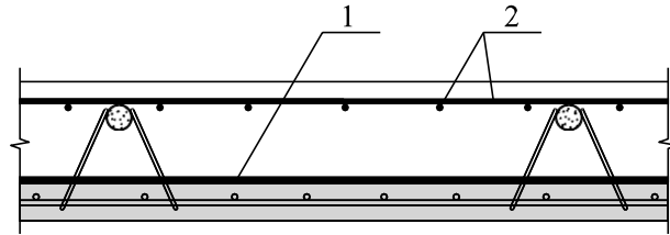
图 5.2.6 叠合层内钢筋
