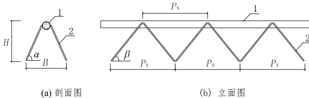
图 1 灌浆钢管桁架
