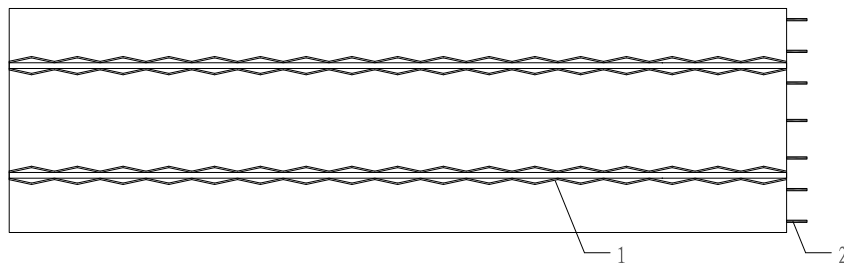
(a) 钢管桁架预应力混凝土预制底板（俯视图）
