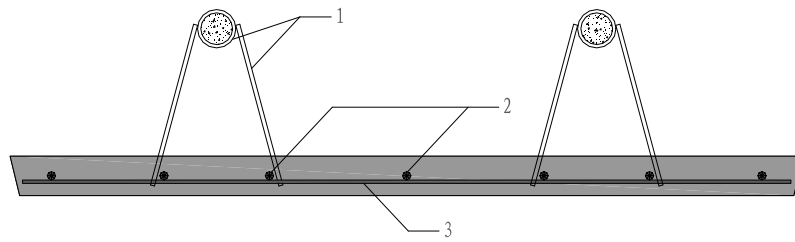
(b)横剖面示意图
