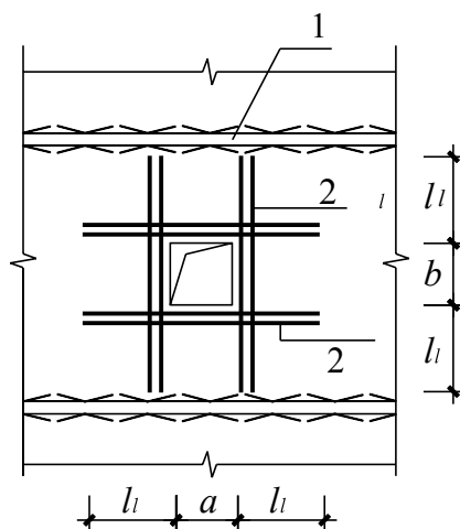
图5.2.9 预制底板开洞加强措施
